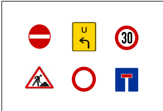
Verkehrsschilder - diverse
